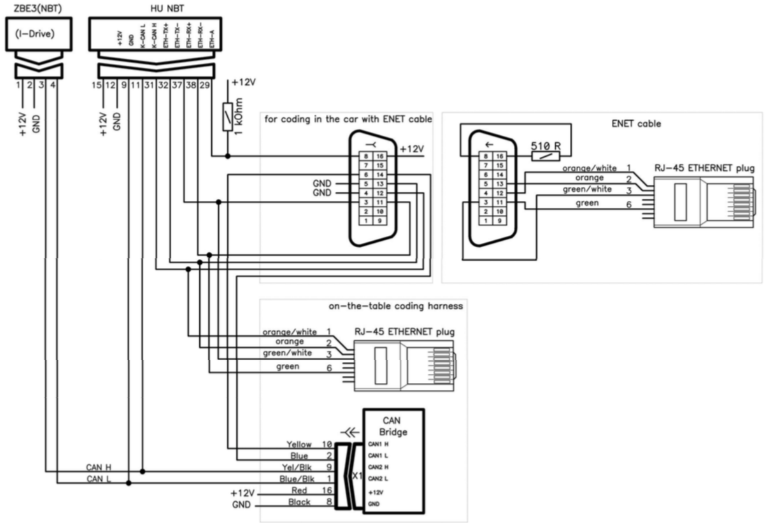
NBT ETHERNET WIRING FOR CODING
